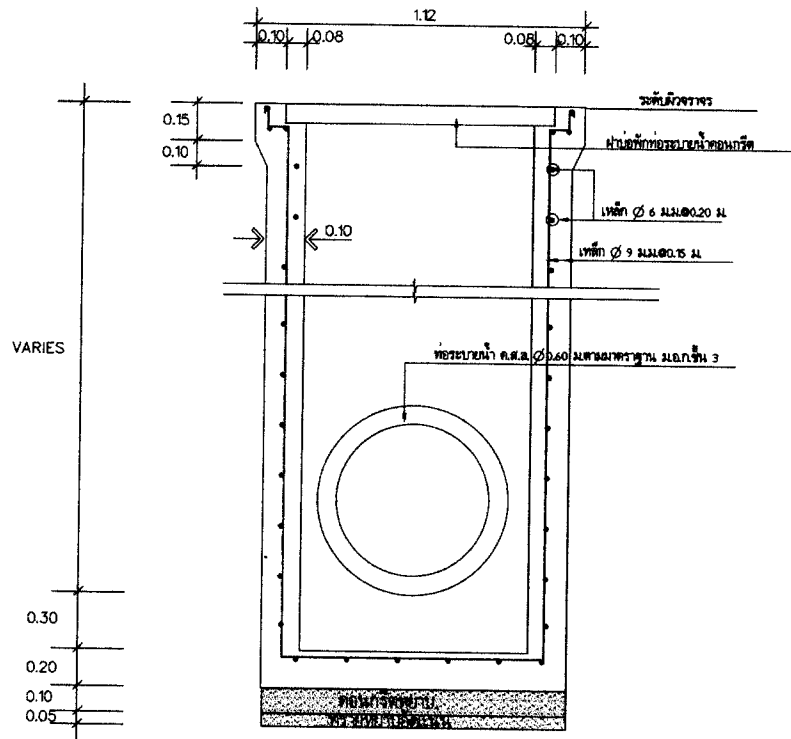
รูปตัดท่อน้ำแนว A-A
