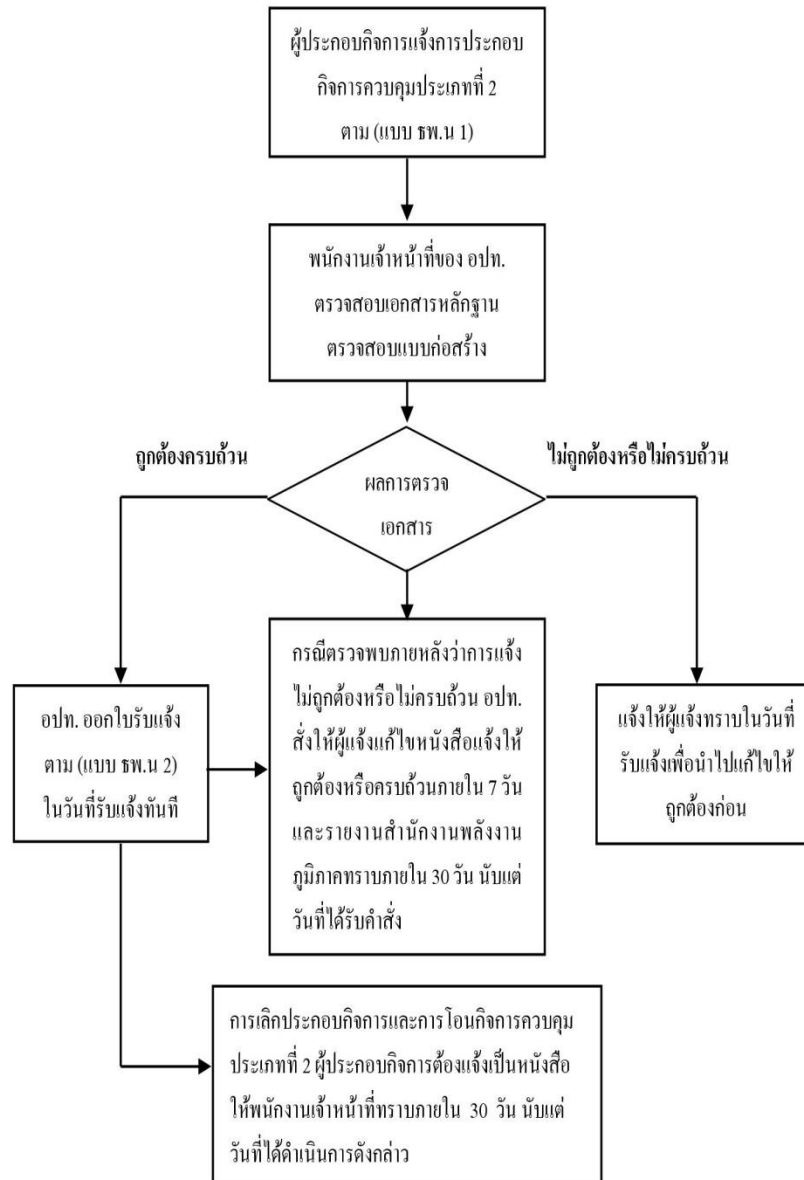
รูปที่ 3-1 แผนภูมิแสดงขั้นตอนการแจ้ง การพิจารณาการแจ้งการเลิกประกอบกิจการและ การโอนกิจการของผู้ประกอบกิจการควบคุมประเภทที่ 2 (ป้มาถึงलयริมถนน ขนาดเล็ก ป้มหลอดแก้วมือหมุน และสถานีบริการทางนำขนาดเล็ก)
