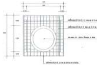
แบบขยายเหล็กปากท่อระบายน้ำ : No Scale
